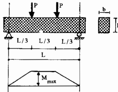
تصویر ۲-۴: تیر بتنی جهت آزمایش تعیین مقاومت کششی ناشی از خمش
