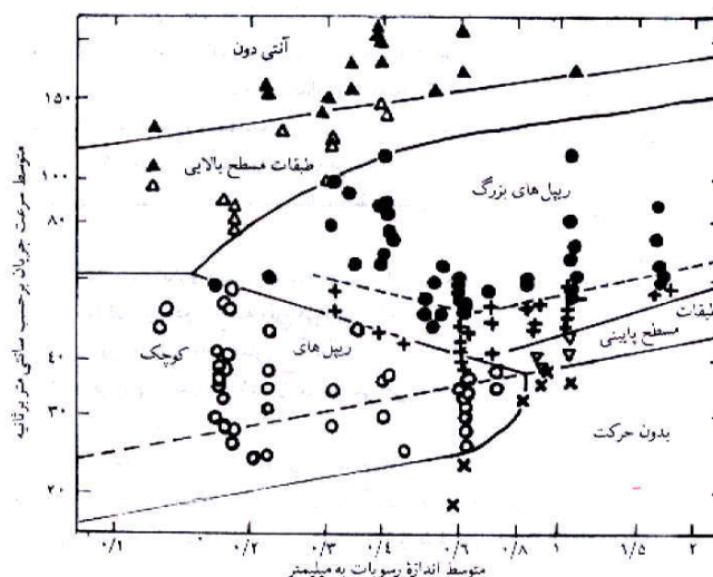
— دیاگرام ارتباط بین اندازه دانه و سرعت جریان در حالتی که عمق آب بین ۱۸ تا ۲۲ سانتی متر بوده است. دایره های توخالی، ریپل مارک های کوچک؛ علامت به علاوه ریپل های بزرگ دو بُعدی (مگاریپل و امواج ایستاده)، دایره های توپر، ریپل های بزرگ سه بُعدی (مگاریپل ها و دون ها)؛ مثلث های توخالی، طبقات مسطح بالایی؛ مثلث های توپر، آنتی دون (دون برگشتی)؛ مثلث های توخالی معکوس، طبقات مسطح پایینی؛ و علامت x، بدون حرکت بودن دانه های رسوبی (اقتباس از هارمز و دیگران، ۱۹۸۲).
