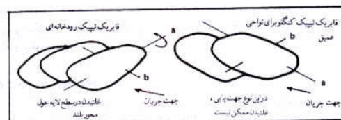
اختلاف بین فابریک دانه های درشت در کنگلومراهای رودخانه ای و کنگلومراهای تواسی که دانه های درشت آنها در اثر حرکت مجدد رسوبات به توسط جریانهای توربیدی تشکیل شده اند (قتاس از واکر، ۱۹۸۴).
