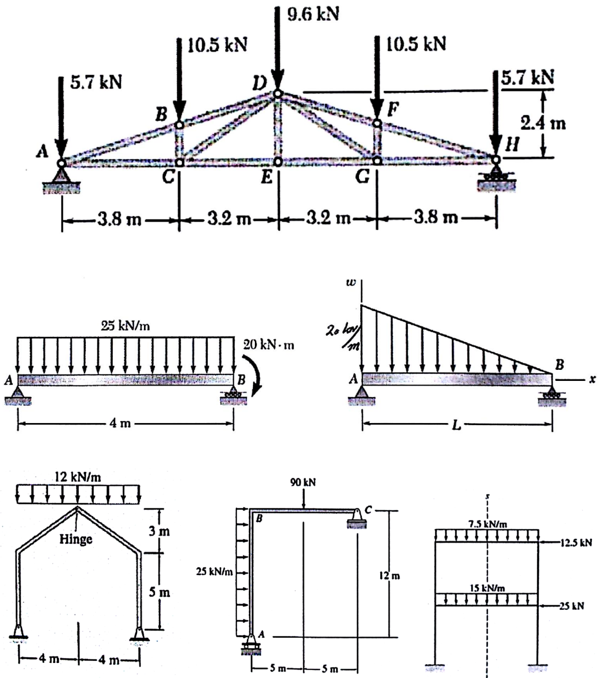
شکل (۲-۱): انواع بار از لحاظ نحوه اثر (متمرکز، گسترده و ...)
