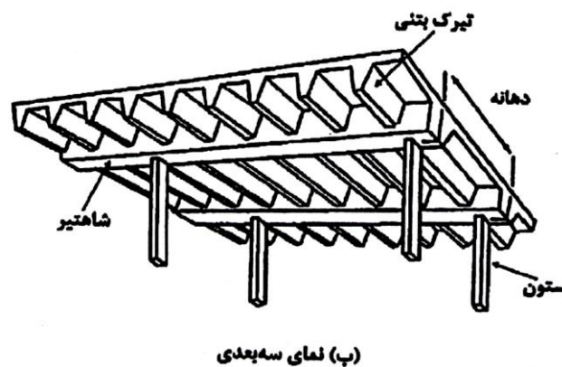
شکل (۲-۱۲): سقف دال تیرک‌دار
