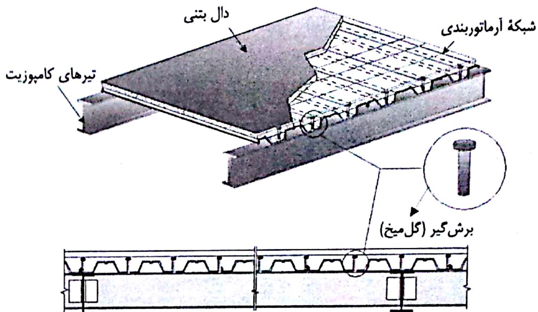
شکل (۲-۱۴): سقف کامپوزیت عرشه فولادی
