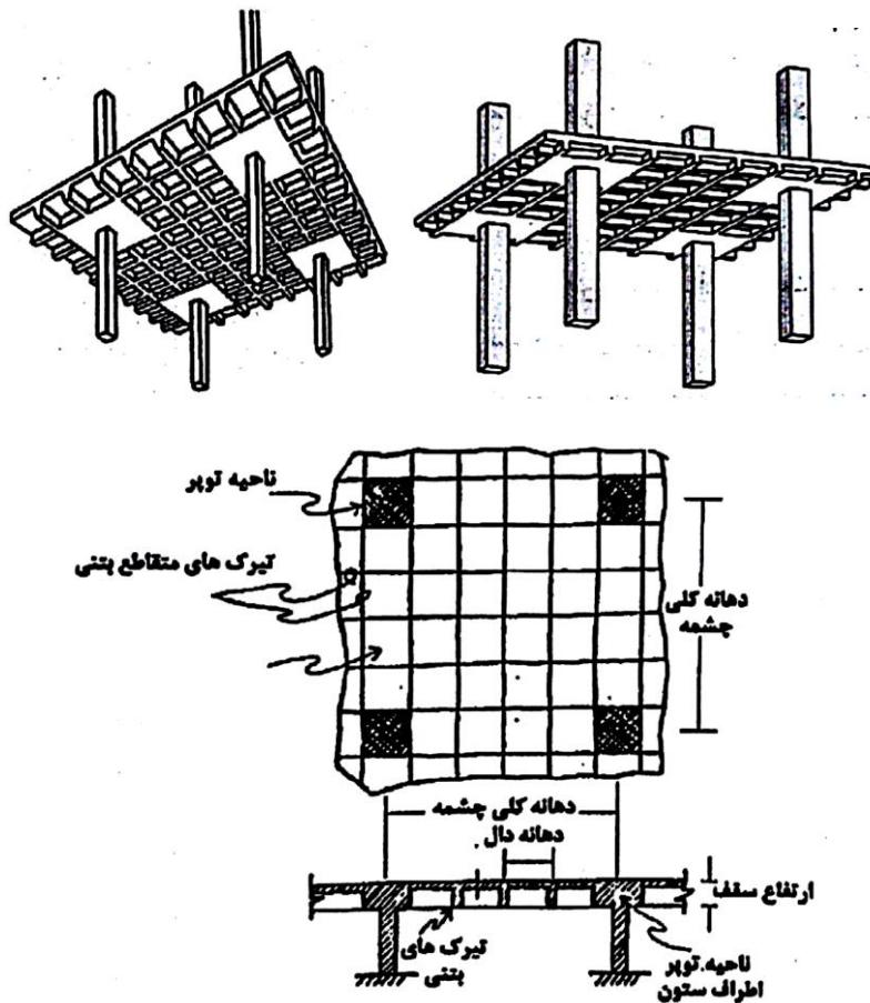
شکل (۲-۲۰): دال دو طرفه‌ی مجوف
