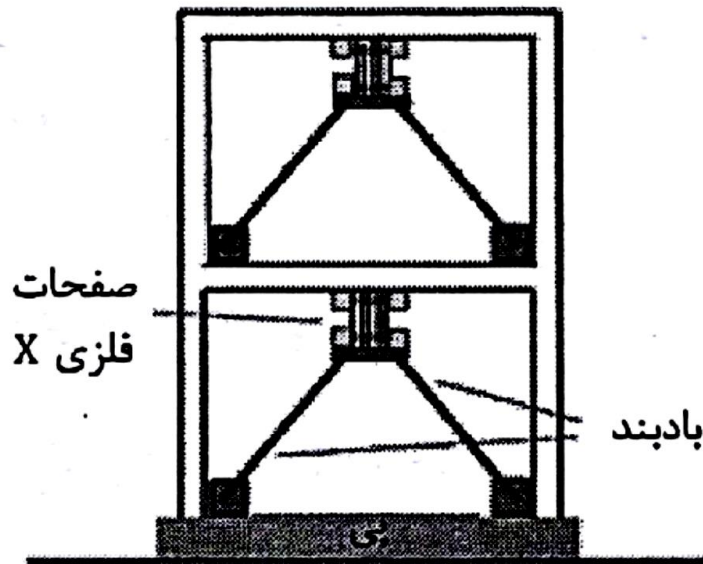
شکل (۹-۷): نحوه استقرار میراگر X-ADAS در قاب
