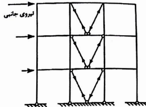
شکل (۲-۲۸): مهاربند ۷ یا ۸
