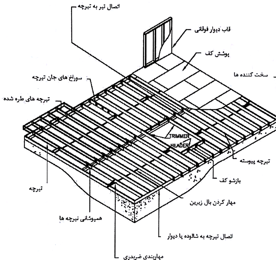
شکل (۴-۱۶): شکل کلی سیستم کف
