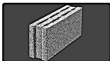
دیواری توخالی (سه جداره) Size: 49×12×20 Max. Weight: 9.2 kg Sound Resistance: 49 db
