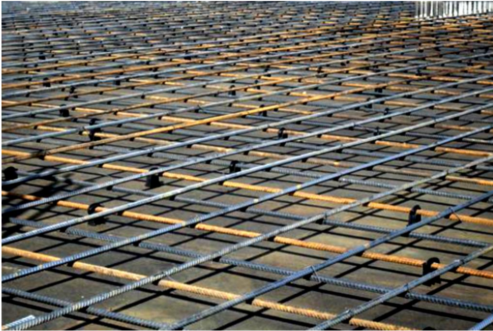
شکل (۶-۷): آرماتورگذاری سفره تحتانی در سقف یوبوت
