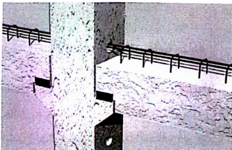
شکل (۵-۷): اتصال تیرهای کوتاه به ستون در طبقات
