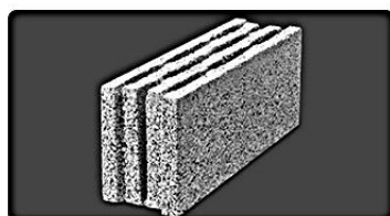
دیواری توخالی (چهار جداره) Size: 49×14.5×20 Max. Weight: 11.2 kg Sound Resistance: 50 db
