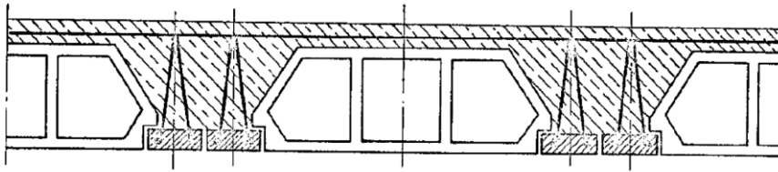
شکل (۲-۱۰-ب): سقف با تیرچه‌های مضاعف
