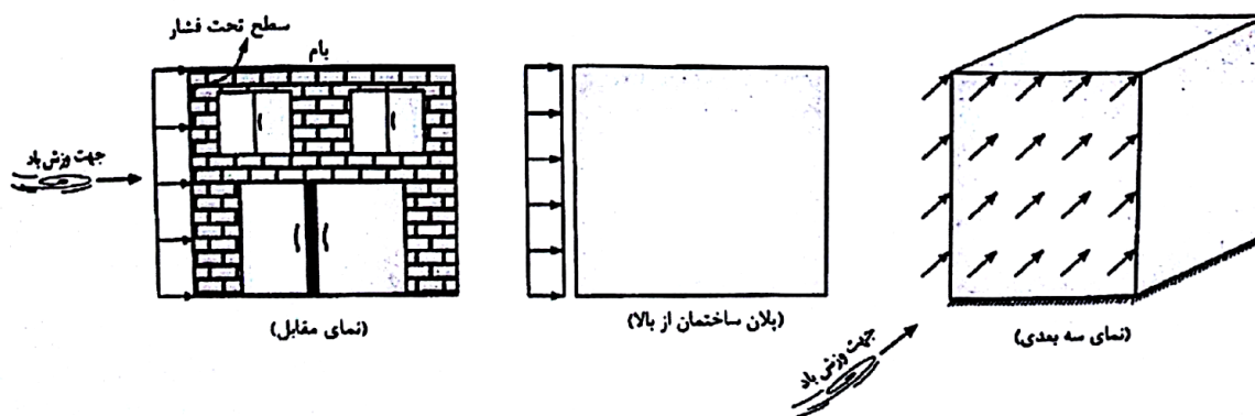
شکل (۱-۶): ایجاد فشار در سمت رو به باد
