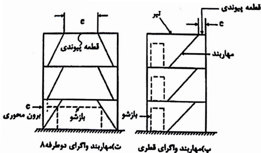
شکل (۲-۲۹): مهاربند واگرا
