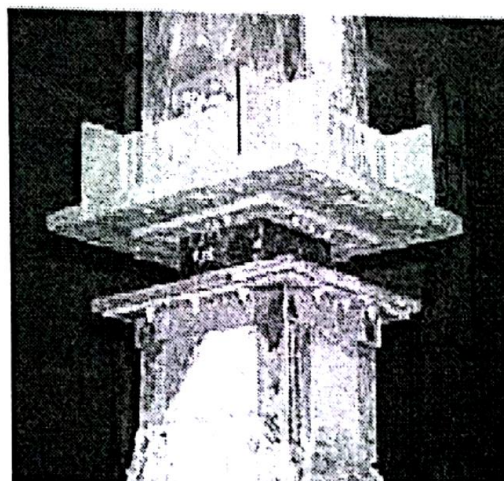
شکل (۹-۱۵): جداگر لرزه‌ای
