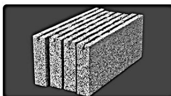
دیواری توخالی (هشت جداره) Size: 49×25×20 Max. Weight: 17 kg Sound Resistance: 54 db
