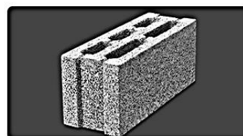
دیواری توخالی ته پر (سه جداره) Size: 49×17.5×20 Max. Weight: 12 kg Sound Resistance: 50 db
