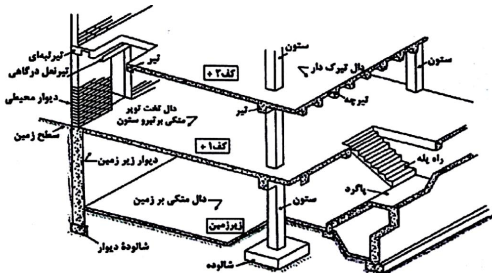
شکل (۱-۳): اجزایی از ساختمان که در بار مرده مشارکت دارند
