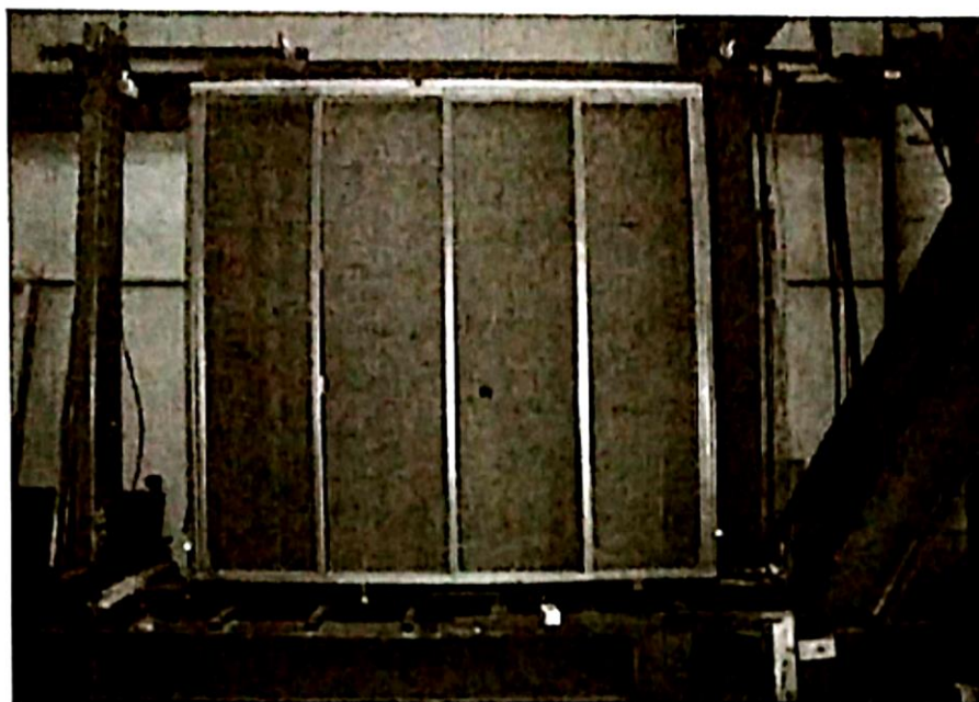
شکل (۴-۳۰): سیستم دیوار برشی با پوشش دیوارهای چوبی استاندارد
