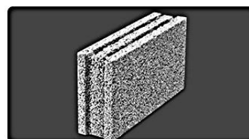
تیغه ای توخالی ته پر (سه جداره) Size: 49×10×20 Max. Weight: 7.5 kg Sound Resistance: 47 db
